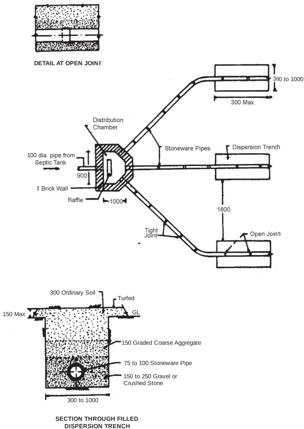
Fig. 19.18 : Dispersion Trench
