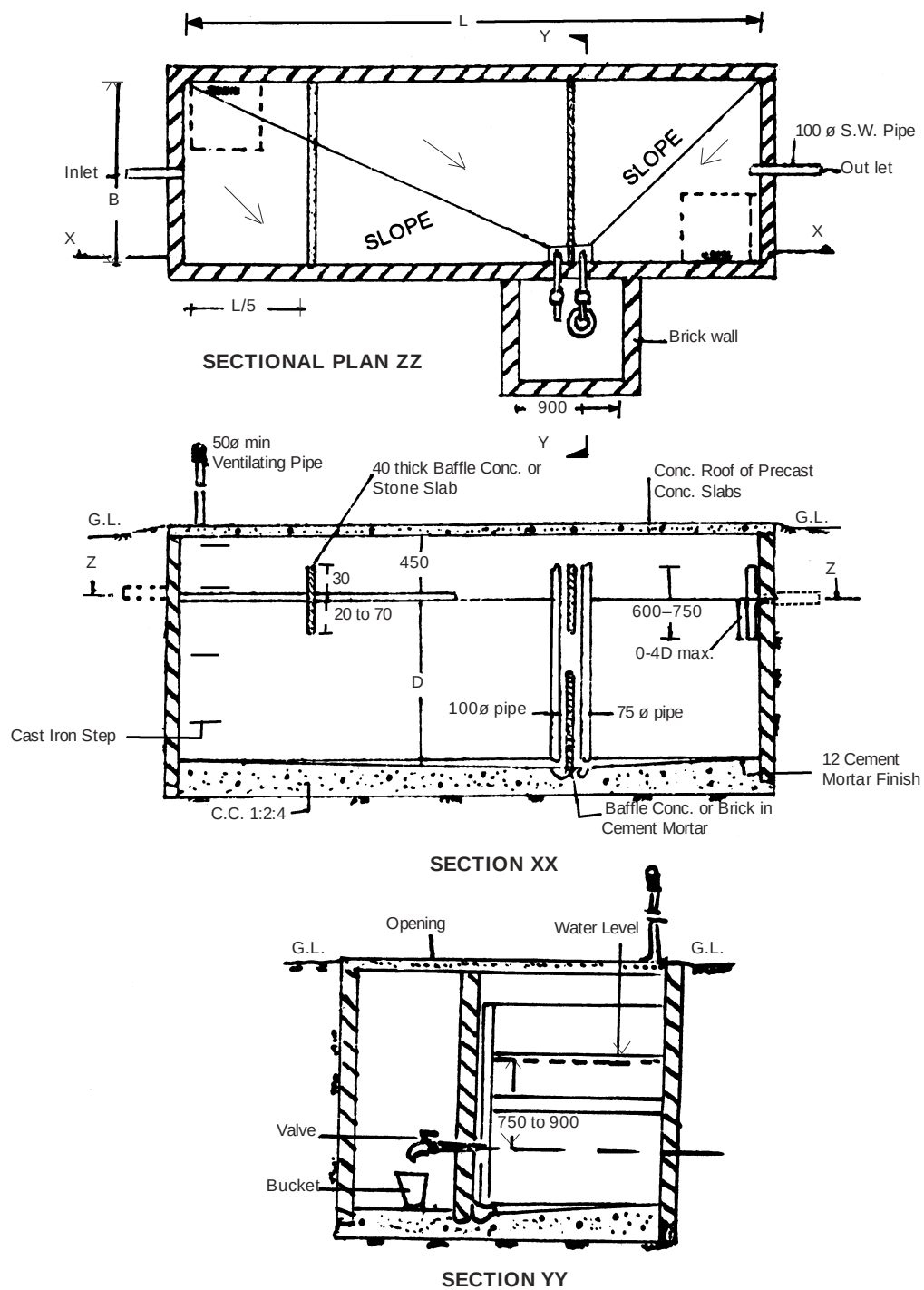
Fig. 19.15 : Septic Tank
